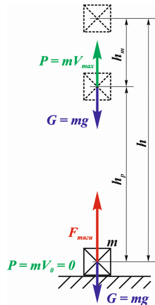
Рис 4.1 Расчётная схема подъёма тела массой m на высоту h
